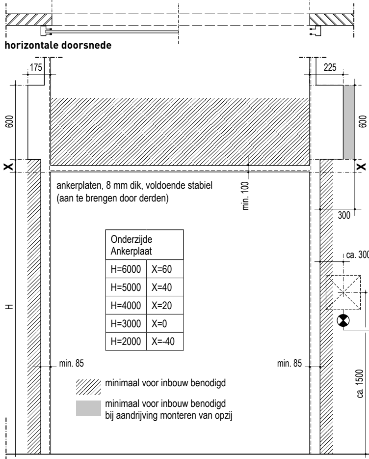
bouwkundige voorzieningen
