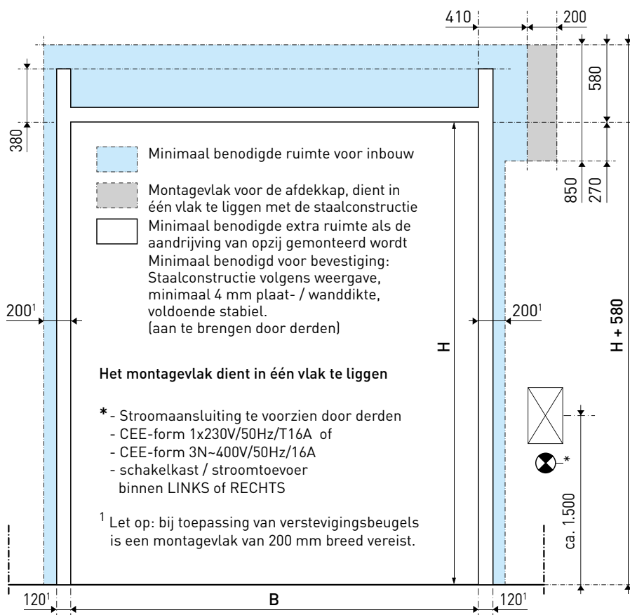
[ Vooraanzicht ]
