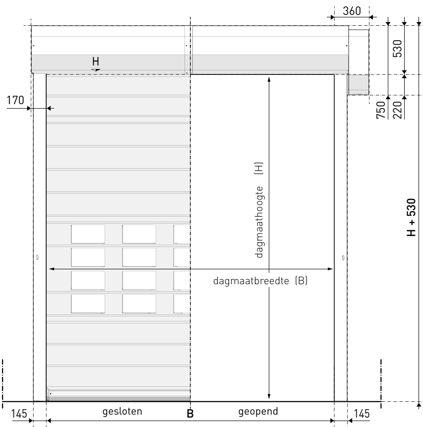
[ Vooraanzicht ]
