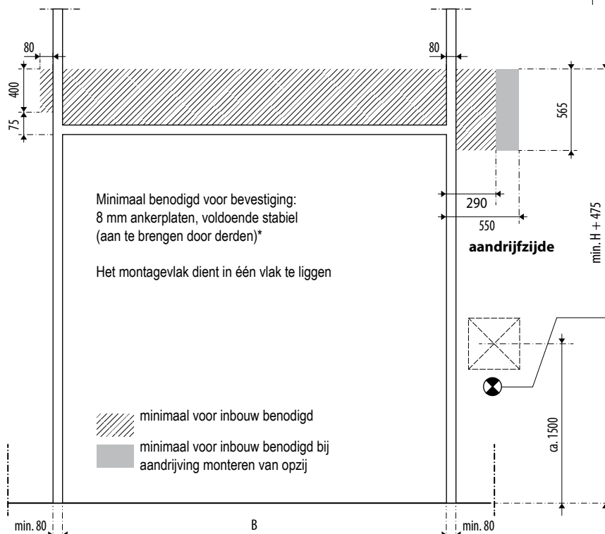
doorsnede A
