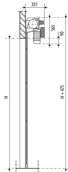
dwarsdoorsnede
