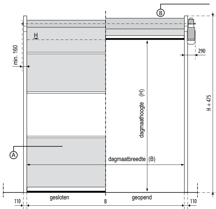
vooraanzicht
