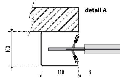
dwarsdoorsnede
