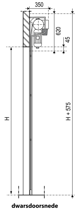
dwarsdoorsnede
