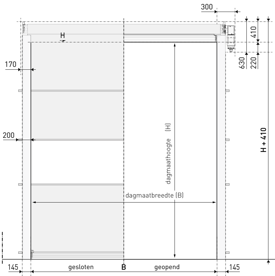
[ Vooraanzicht ]
