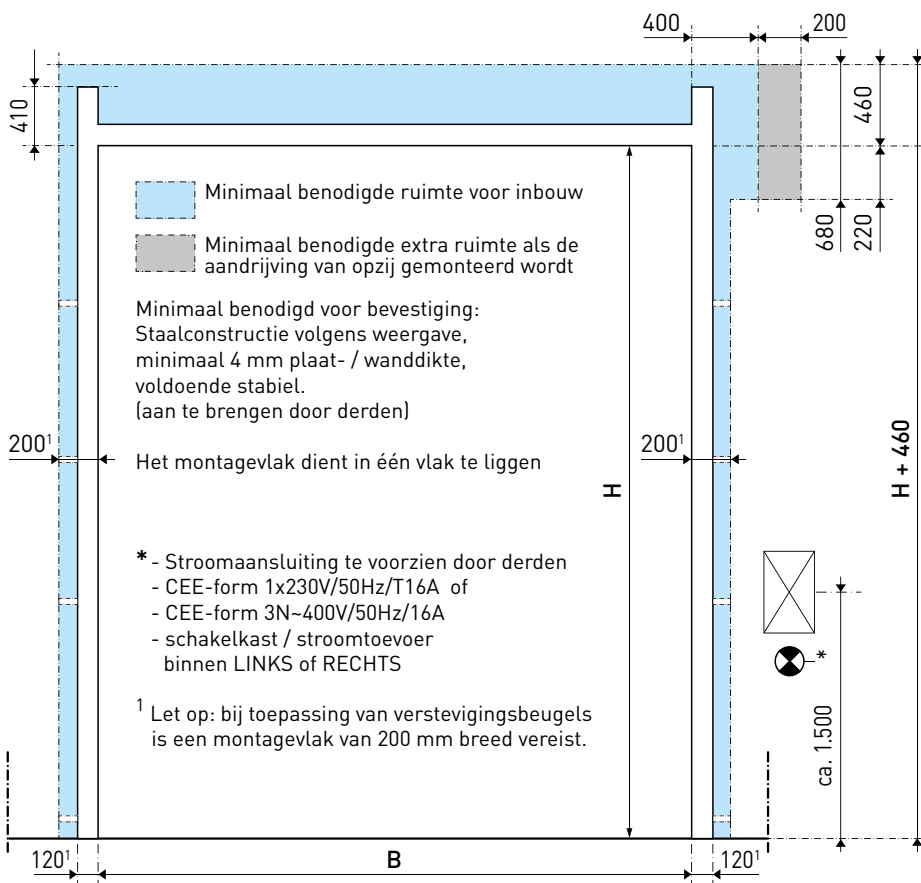
[ Vooraanzicht ]
