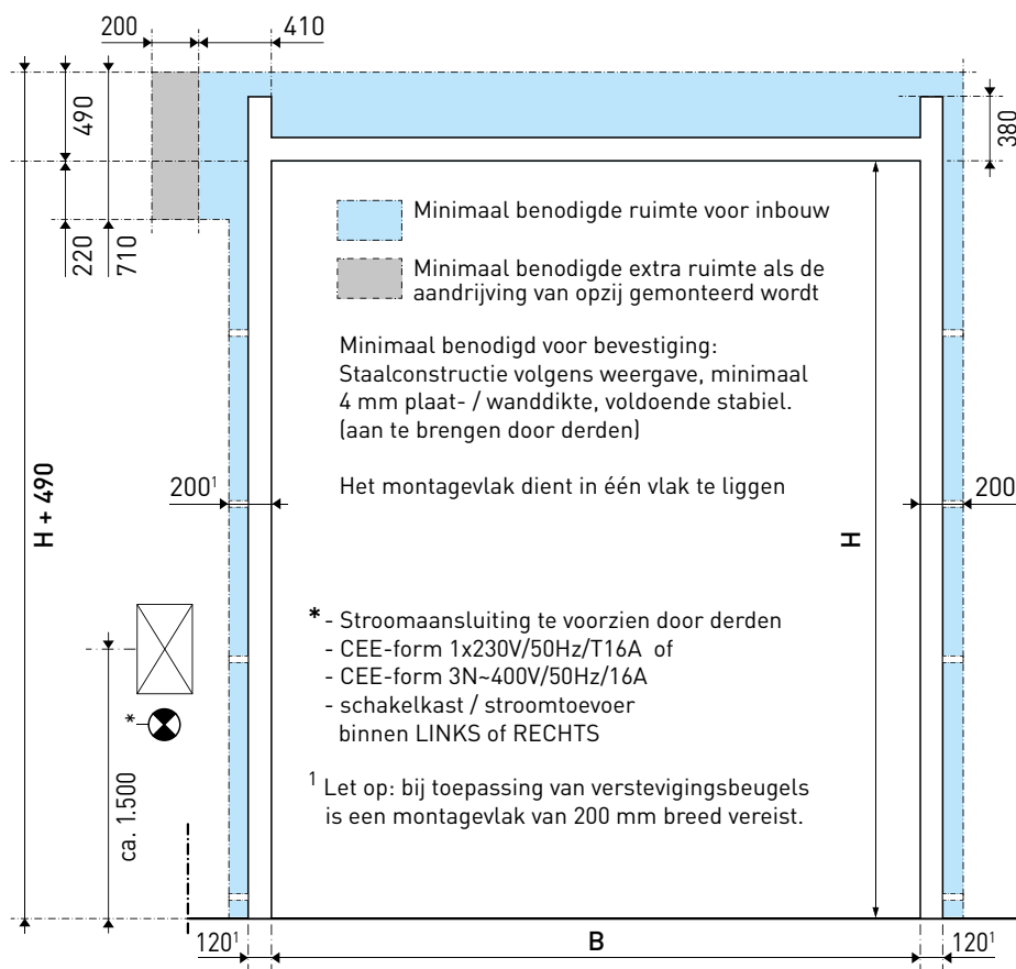
- [ aandrijfszijde ]
