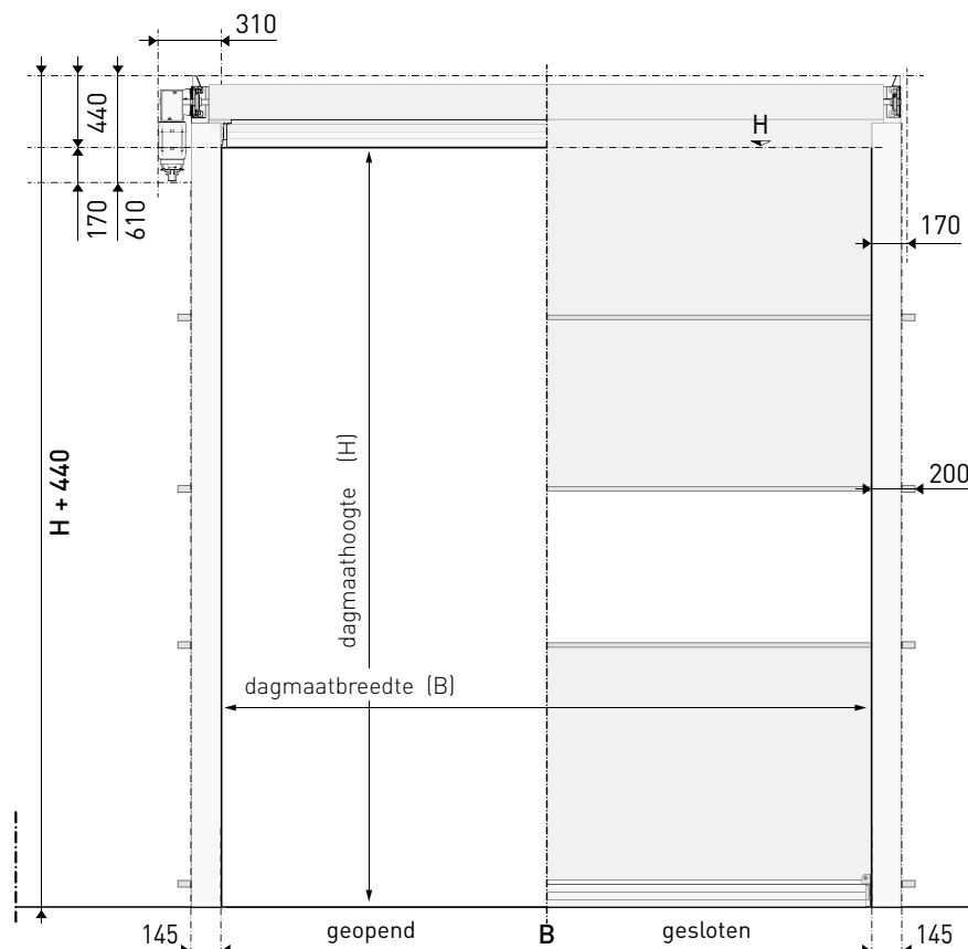
- [ aandrijfszijde ]
