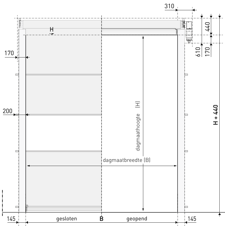
[ Vooraanzicht ]
