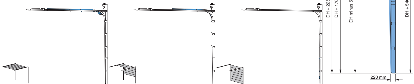
Verloop kabel en deurblad in verschillende openingsstadia
