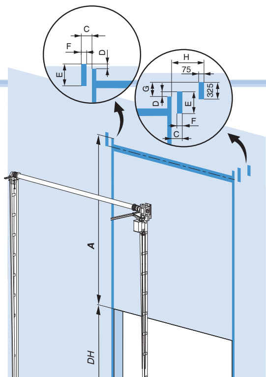
deurbladoppervlak < 35 \text{ m}^2 FLS Veerloze sectionaaldeur
