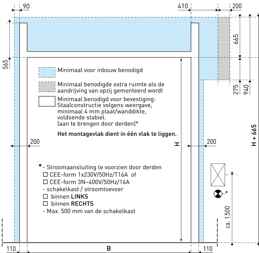
[ Vooraanzicht ]
