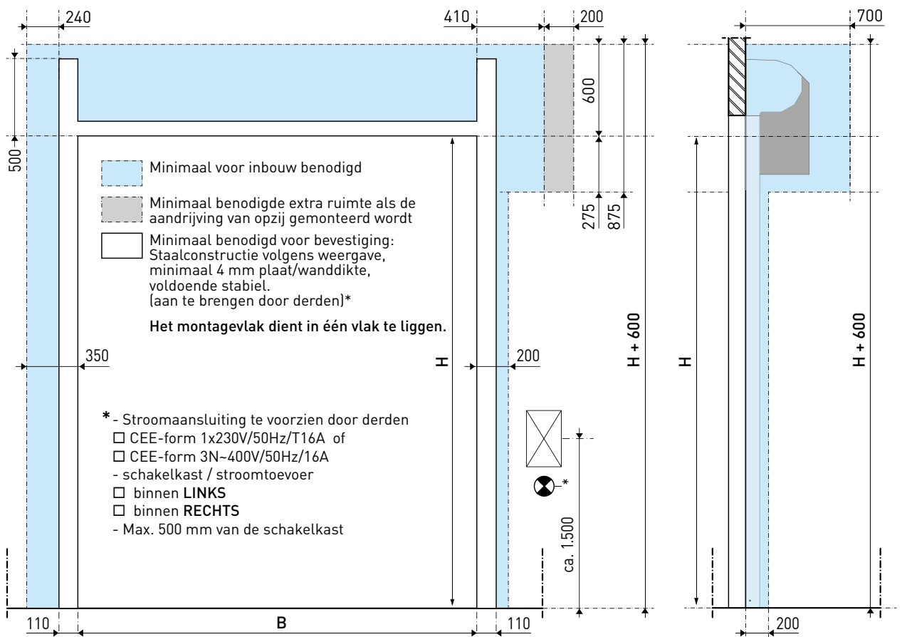
[ Vooraanzicht ]
